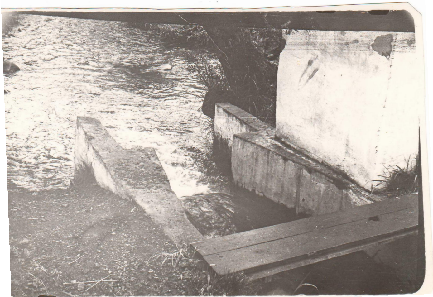
Гидрометрический лоток на ручье Коркина, с Паратунка
